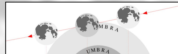
Přiblížení polostínového zatmění 5. června 2020. (zdroj: www.astro.cz )
