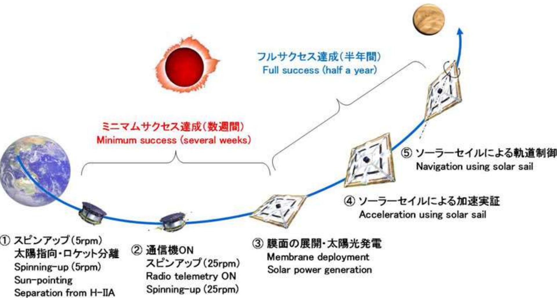
ミッションシーケンス Mission sequence
